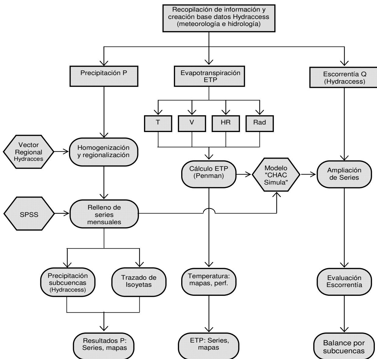
Figura 3.2: Esquema metodológico del Balance Hídrico Microregional
