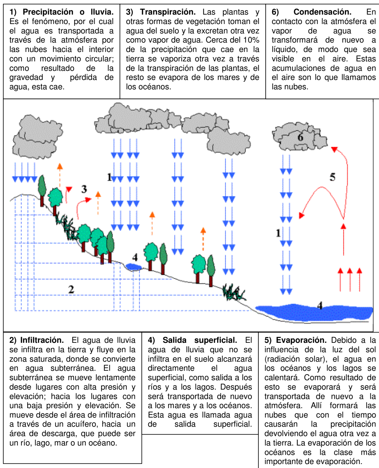
Figura 3.1: Ciclo hidrológico
