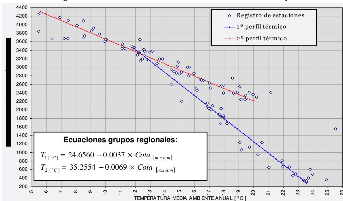
Figura 5.1: Perfiles térmicos - Cuenca Alta del río Pilcomayo
