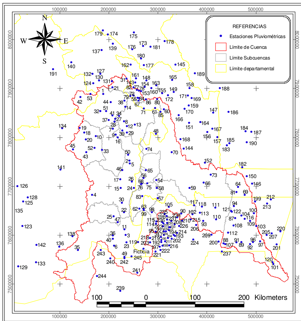
Figura 4.2: Ubicación de estaciones pluviométricas
